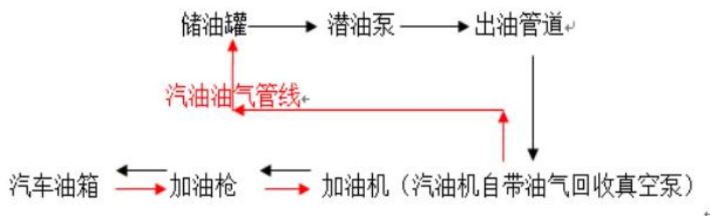
图 2-5 汽油加油流程框图
