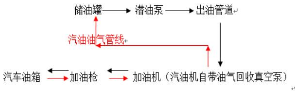
图 2-5 汽油加油流程框图
