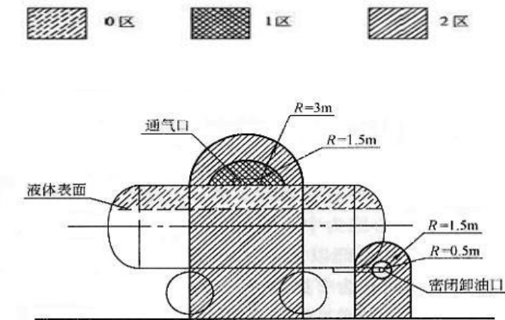
附图 2 油罐车和密闭卸油口爆炸危险区域划分
