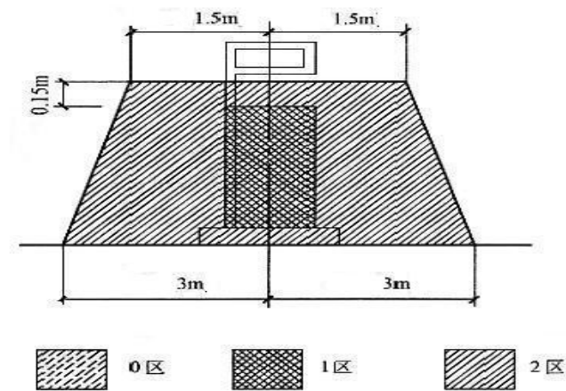
附图 1 汽油加油机爆炸危险区域划分
